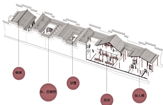
图 3 胜利街 242 号轴测图 (来源: 自绘)
